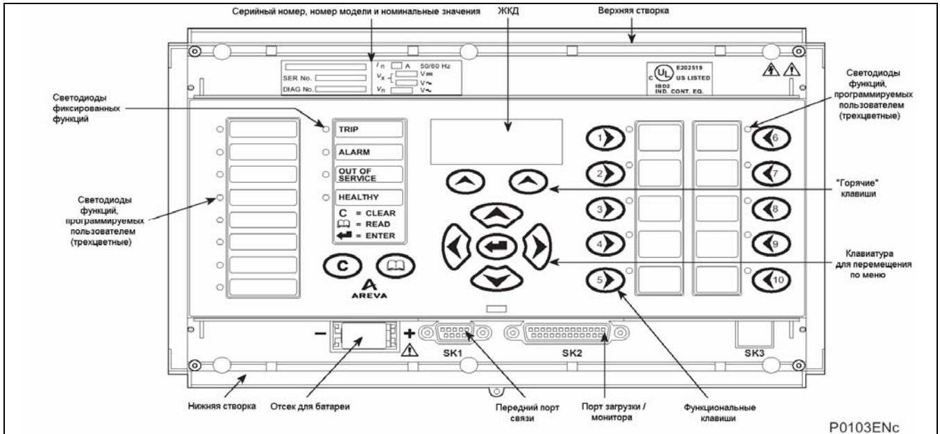
Рисунок 2: Вид передней панели реле (P345)
