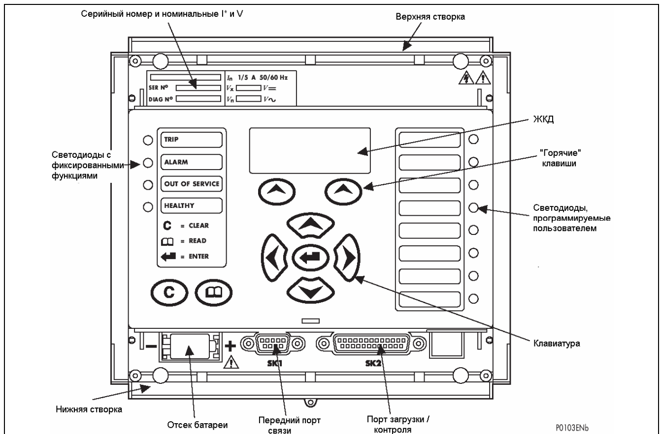
Рисунок 1: Вид передней панели реле (P342/3/4)
