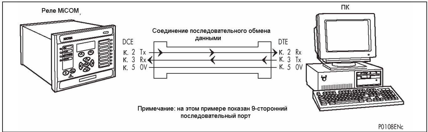
Рисунок 8: Соединение реле с ПК
