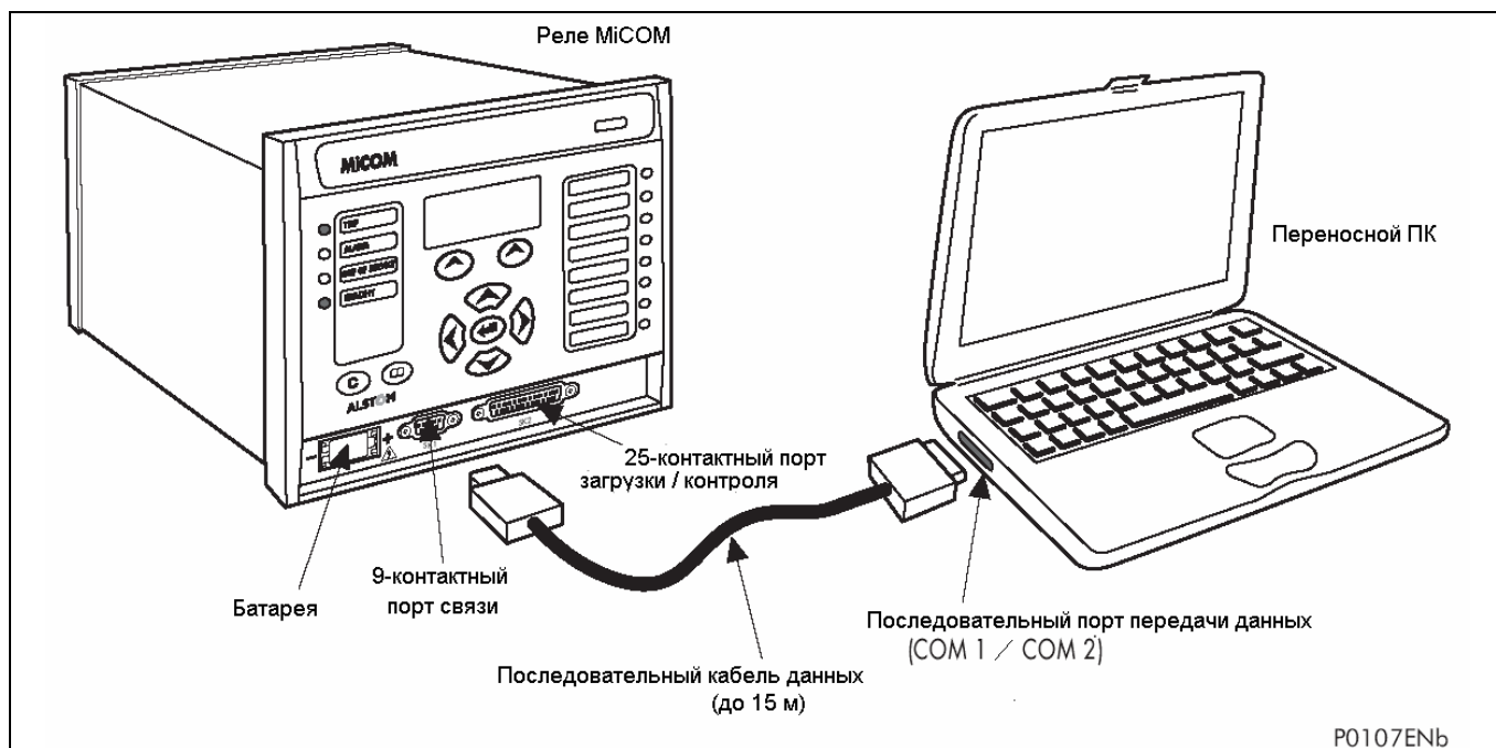
Рисунок 7: Подключение переднего порта реле
