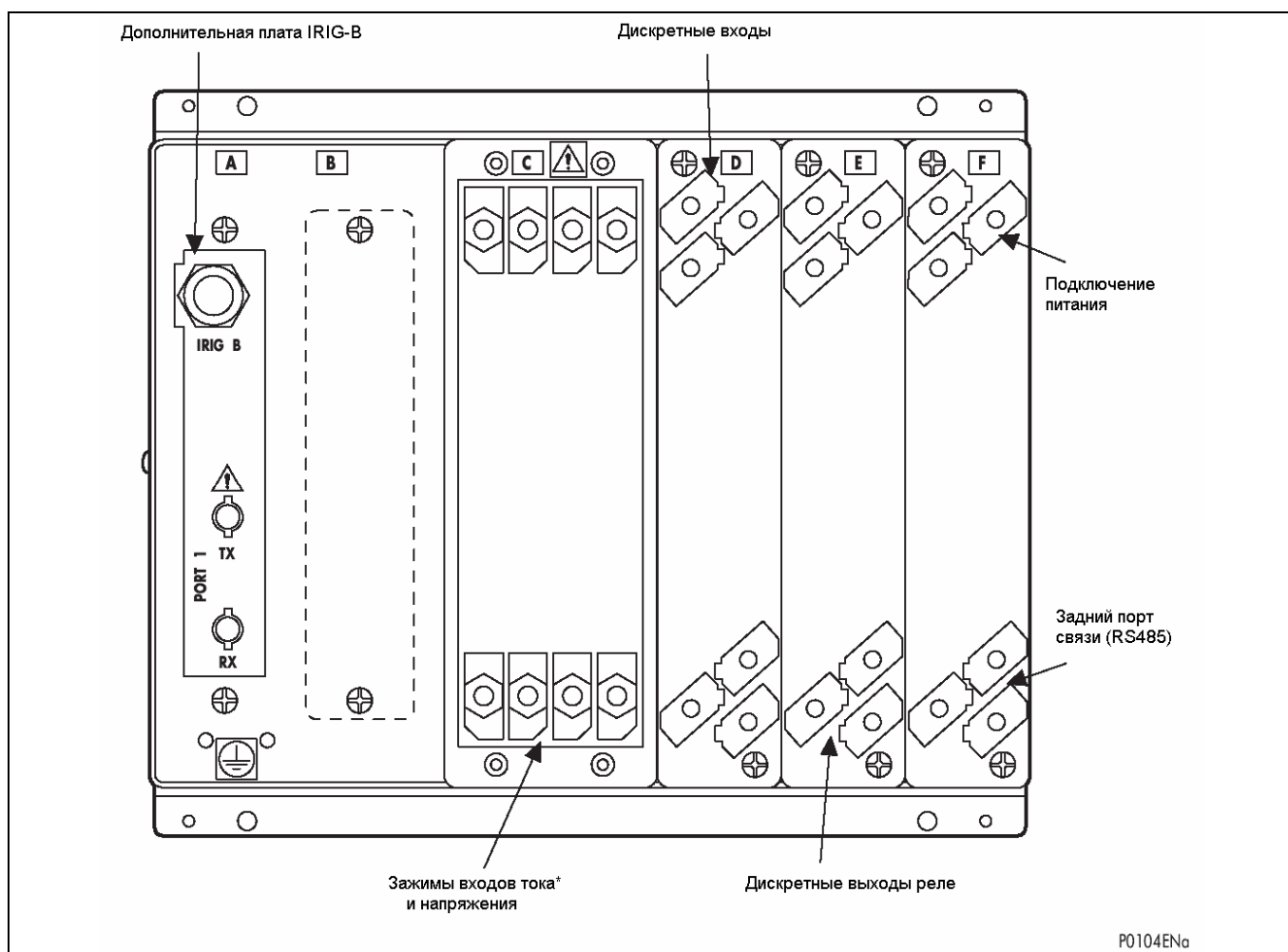
Рисунок 3: Вид задней панели реле
