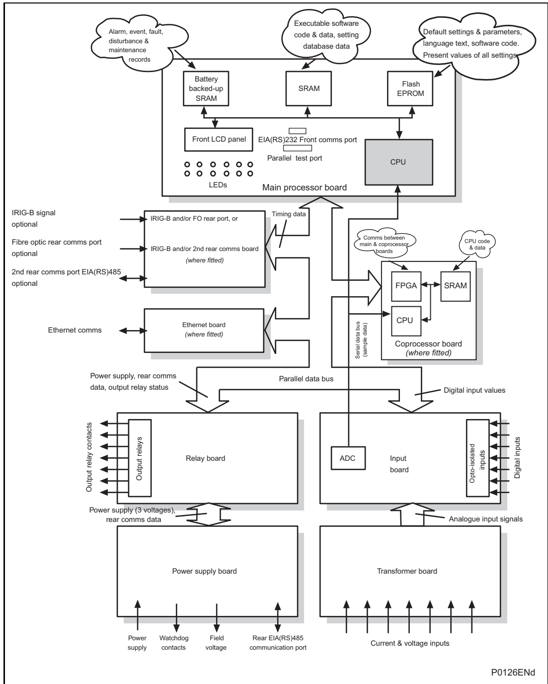
Рис 1: Модули терминала и потоки информации
