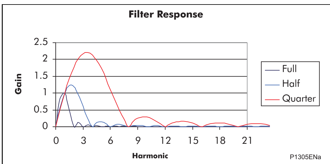
Рис 7: Частотные характеристики фильтров
