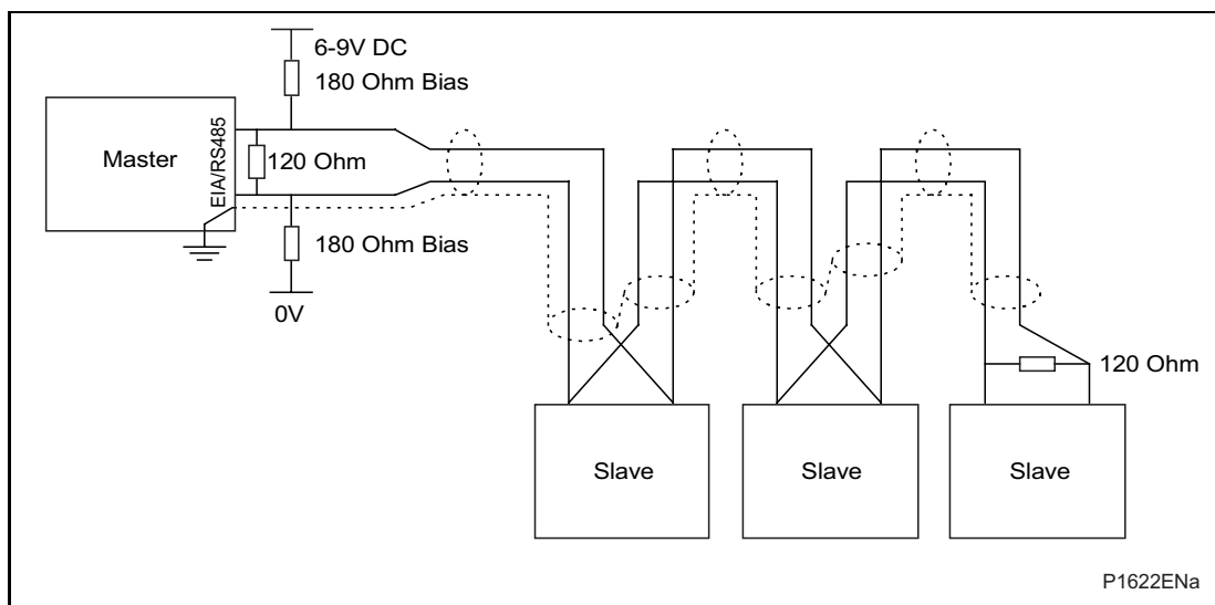
Figure 1: Схема подключения по EIA(RS)485
