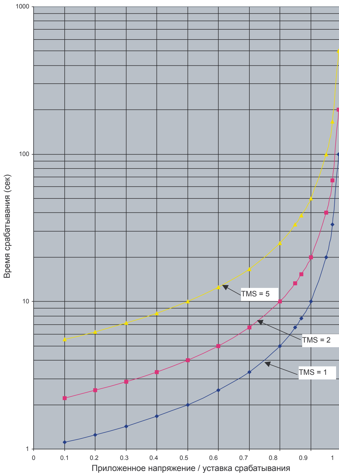
Рис. 1: IDMT характеристики для первой ступени защиты минимального напряжения "V<"
