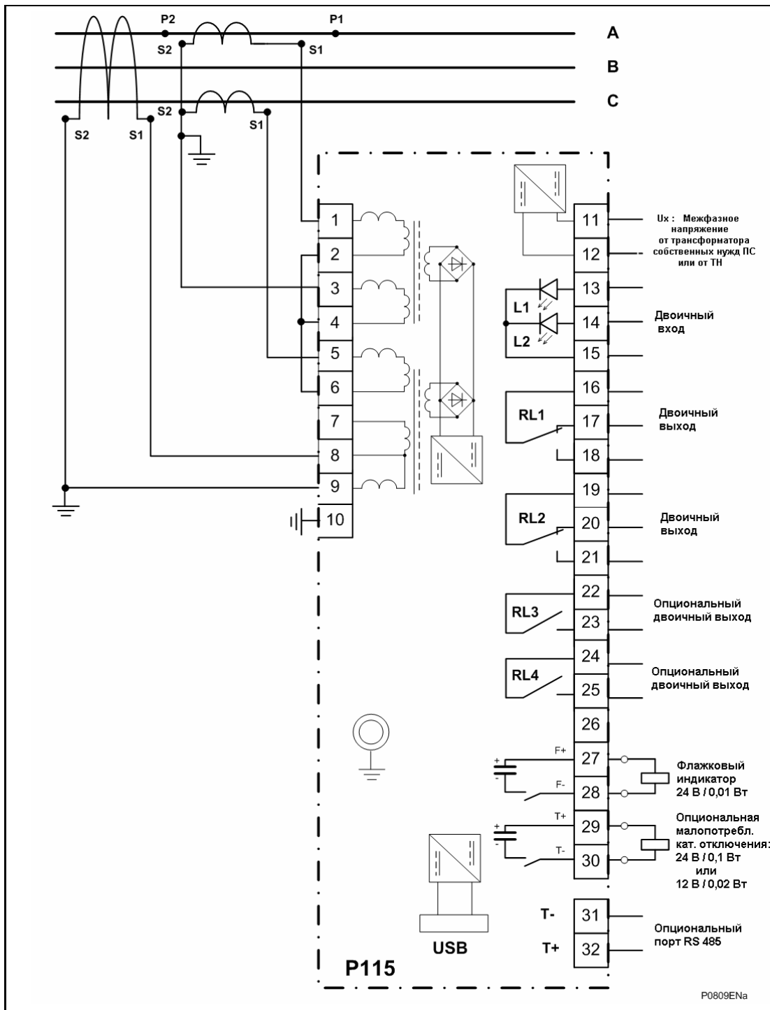
Рисунок 5: Типичная схема подключения с 2 фазными ТТ + ТТо.
