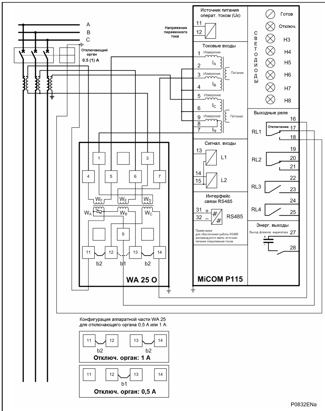
Рисунок 6: Пример схемы подключения устройства P115 с питанием от WA 25 O и при 4-полюсном соединении (A-B-C-N)
