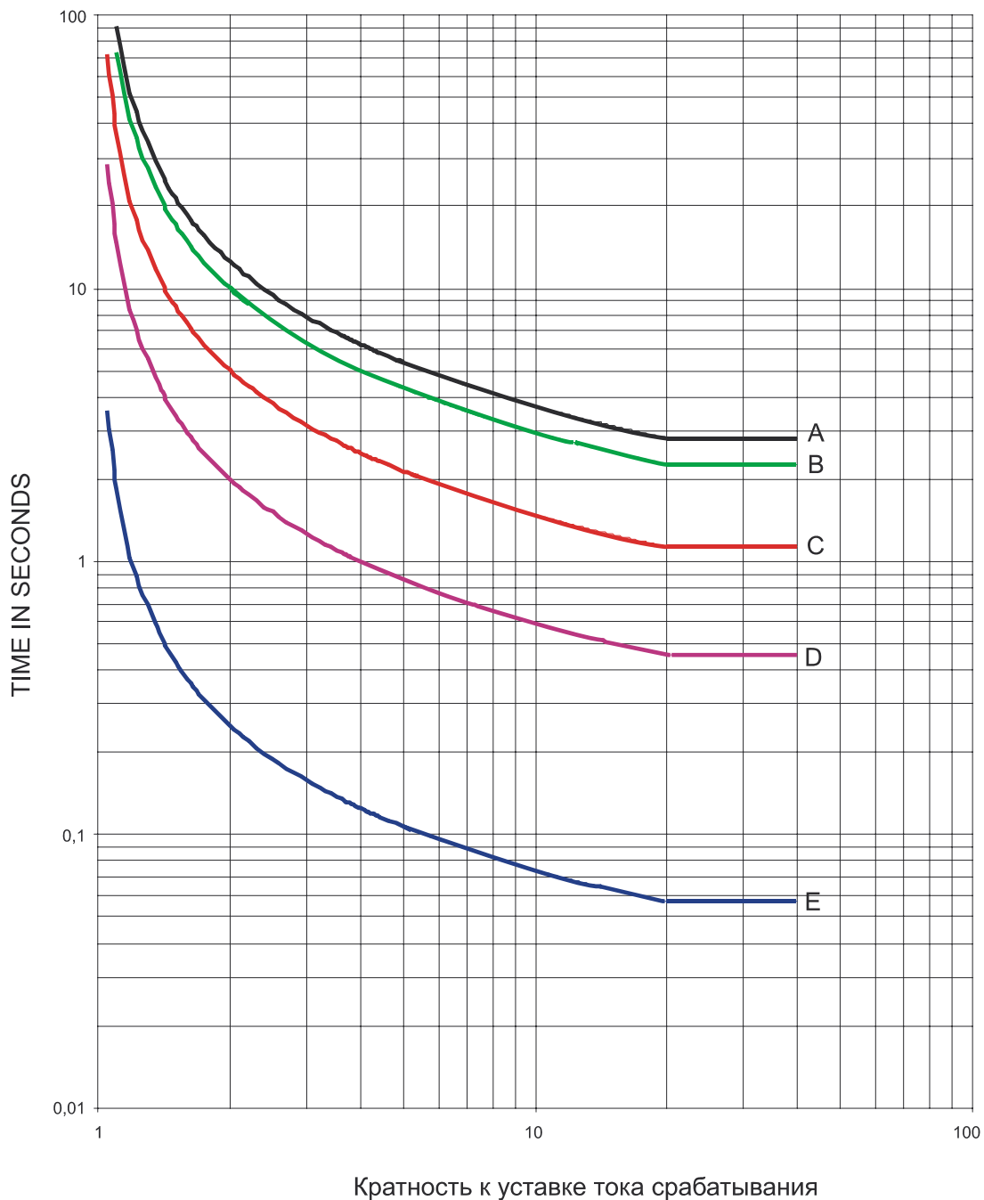
Стандартная инверсная МЭК (IEC)
